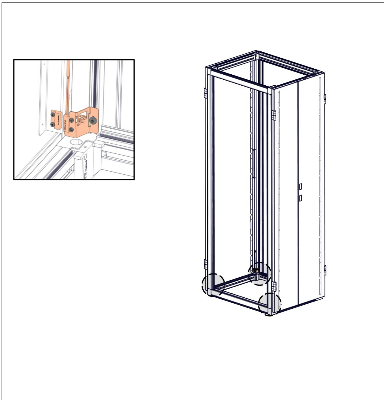
Door Sensor Assembly
