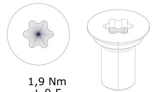
M5 x 10 (T25)
