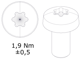
M5 x 10 Metr (T25)
