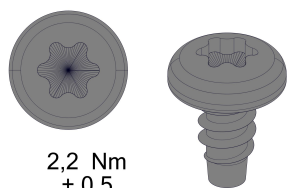
ST 4,8 x 8 (T25)
